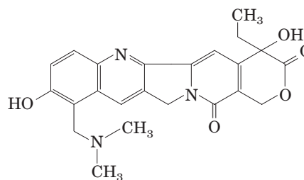
Topotecan
