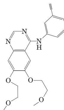
Erlotinib (Tarceva)
