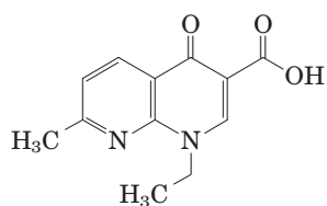
Nalidixic acid
