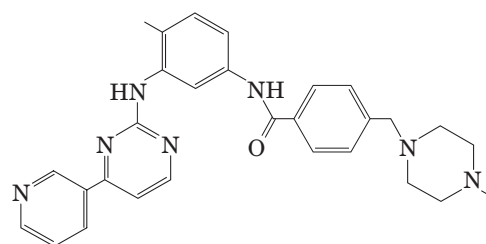
Imatinib (Gleevec)
