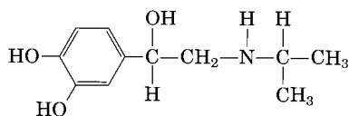
Isoproterenol
